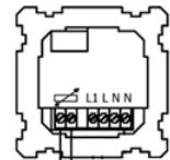
Anschluss Fensterkontakt
