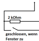
Anschluss Fensterkontakt
